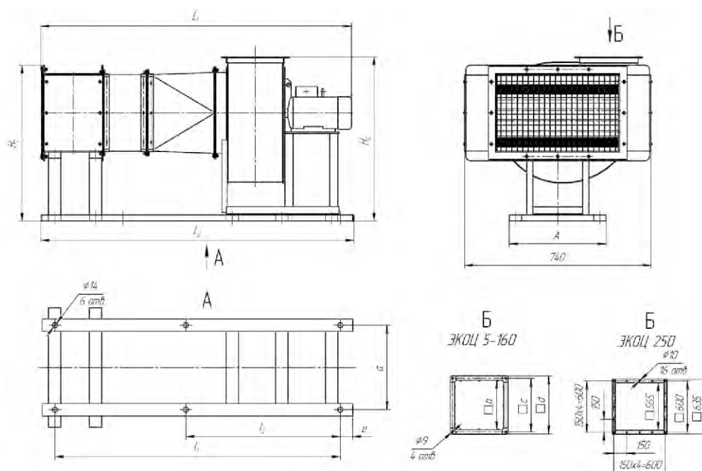
Рис. 42. Габаритные и присоединительные размеры установок ЭКОЦ.
