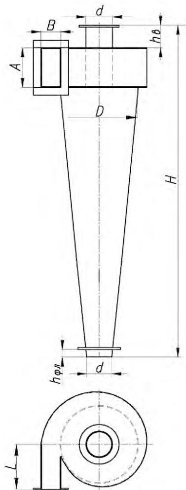
Рис. 13. Габаритные и присоединительные размеры СДК-ЦН-33.
